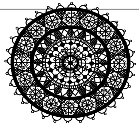
Čipka konstruirana u Geogebri
